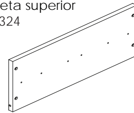
P. Top Drawer Side x6 Barre de tiroir supérieur Barra de la gaveta superior #29085
