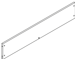
L. Drawer Back x3 Arrière du tiroir Trasera de la gaveta #29138
