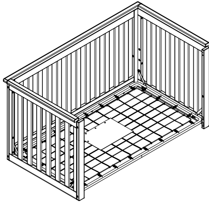
From Section 2 Step 2 monté à l'étape 2 de la section 2 de la sección 2, paso 2
