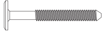
C. M6x50 mm \Phi 17 Head Bolt x 1 Boulon à tête hexagonale \Phi 17 M6x50 mm x 1 Perno de Cabeza \Phi 17 M6x50 mm x 1
