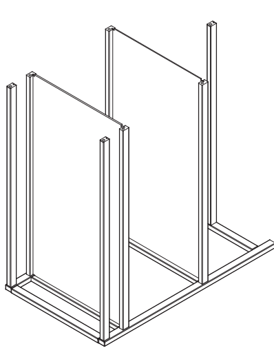
From Step 2 À partir de l'étape 2 Desde el paso 2
