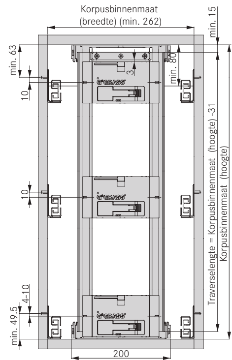
Draagprofielhouder boven/onder
