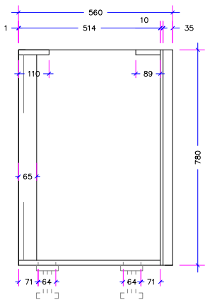
HOEKONDERKAST 780 / 1000 / 560 / 18 t.b.v. LeMans II 45
