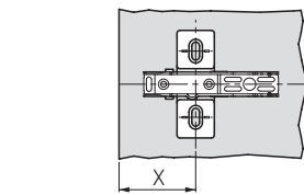
Maatvoering voor kruismontageplaat Bevestigingsafstand 37
