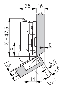
hoogte montageplaat 9
