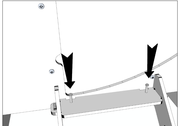
26, Wenn die Leiter in Position ist, stecken Sie die beiden 25mm Gabelkopf Bolzen in die dafür vorgesehenen Löcher.
