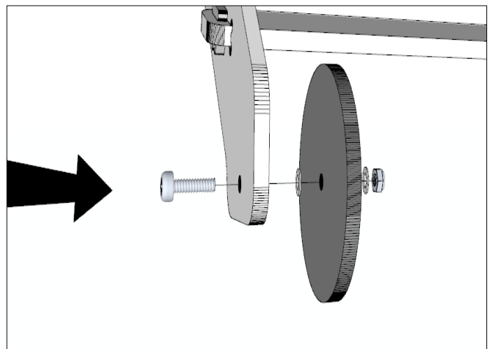
24, Montieren Sie die Pufferscheiben an den Innenwänden der Leiter. Verwenden Sie 1x 30mm Schraube, 1x Standard Unterlegscheibe, dann Pufferscheibe, gefolgt von einer weiteren Standard Unterlegscheibe und 1x Nylon Lock Mutter. Wiederholen Sie den Vorgang für die andere Seite. Ziehen Sie die Schrauben an, bis sich die Pufferscheibe frei drehen lässt.
