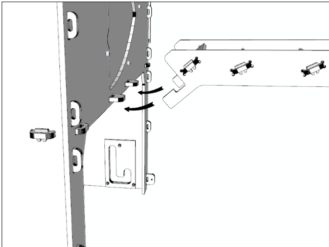
25, Montieren Sie die Leiter, indem Sie den L-förmigen Haken unter den Hühnerstall schieben und die obere Stufe auf die beiden Laschen mit den Löchern setzen.
