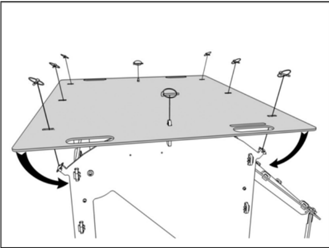
19, Poser et assembler le toit en commençant par le centre et en mettant le côté avec les 3 fentes larges (2 fentes de portage et fente pour la corde de la poignée vers l'avant du poulailler (côté porte)..
