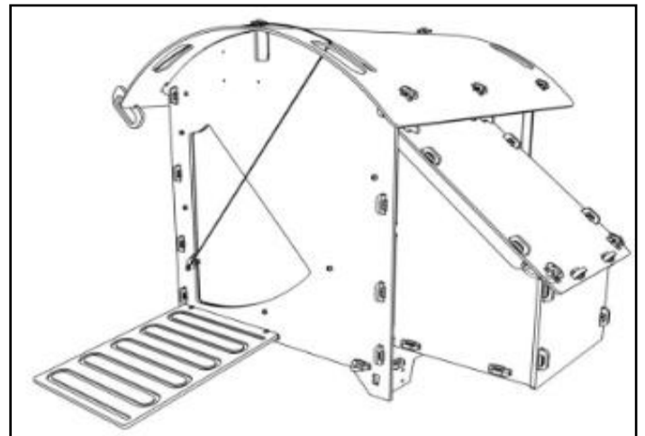
Poulailler Small monté
