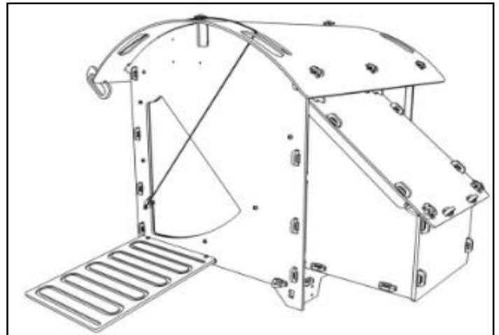
Kompletter kleiner Stall
