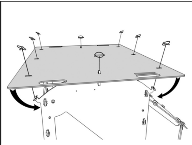
19 , Befestigen Sie das Dach mit Klappsplinten. Befestigen Sie zuerst die Mitte und biegen Sie dann die Seiten über die verbleibenden Laschen nach unten.
