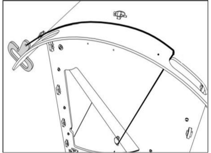
20, PORTE MANUELLE: Raccorder la corde à la bague fendue sur la porte et à l'autre extrémité au trou de la poignée puis faire un nœud pour fixer l'ensemble. La corde doit passer par la seconde fente plus fine située à côté de la fente poignée et une fois ouverte la poignée peut se fixer à l'extrémité du toit pour être maintenue en position porte ouverte.
