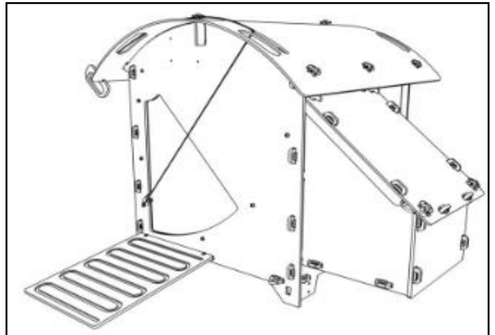
20, PORTE MANUELLE: Raccorder la corde à la bague fendue sur la porte et à l'autre extrémité au trou de la poignée puis faire un nœud pour fixer l'ensemble. La corde doit passer par la seconde fente plus fine située à côté de la fente poignée et une fois ouverte la poignée peut se fixer à l'extrémité du toit pour être maintenue en position porte ouverte.
