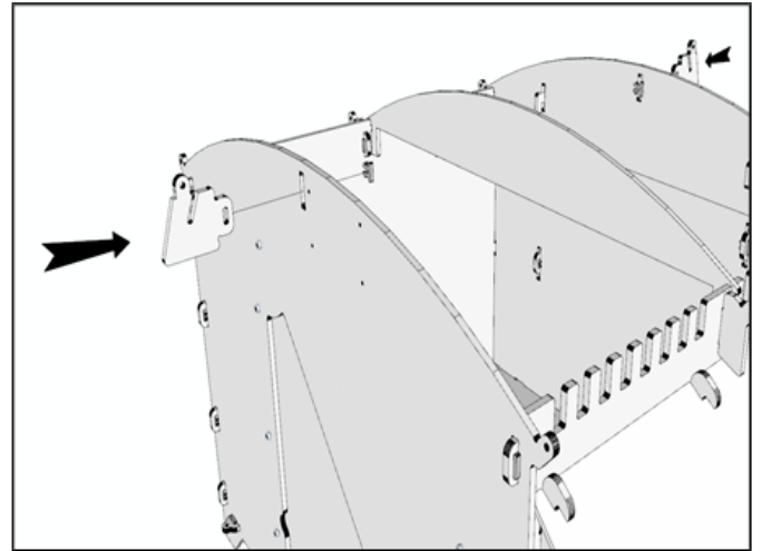
18, Assembler les 2 renforts frontaux et arrière de la toiture sur le mur frontal et le support de toit arrière à l'aide d'un Pi Clip chacun.
