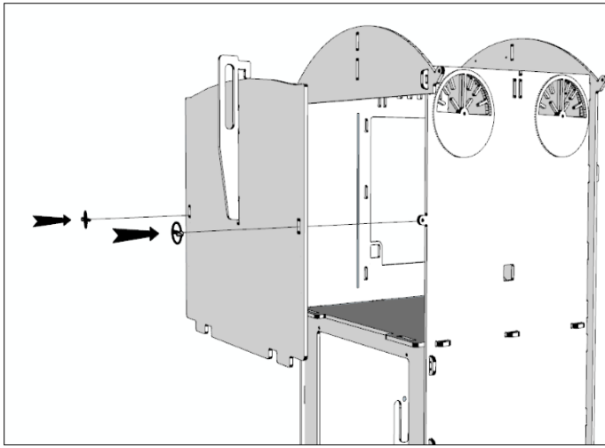
11 , Fixer la porte arrière avec 2 attaches rapides métalliques en insérant les 2 pattes en bas de la porte dans les encoches du plancher puis en poussant la porte, poignée vers le haut, contre le poulailier, puis insérer les 2 attaches rapides de chaque côté. Attention à ne relever qu'un peu l'anneau de attaches rapides afin d'éviter tout pincement.
