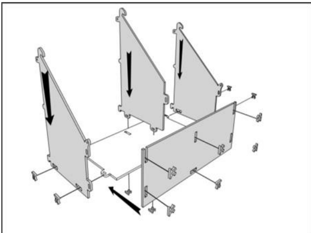
13 , Montez les 2 parois latérales du pondoir et la cloison de séparation sur le plancher du pondoir, puis ajoutez le mur extérieur du nichoir, le tout à l'aide de 12 clips Pi.
