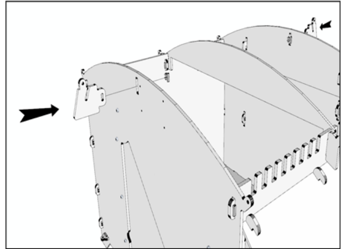
18, Befestigen Sie die Enddachhalterungen mit 1x Pi-Clips an der Vorderwand und der oberen Rückwand.
