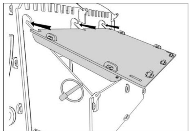
16 , Le toit du pondoir coulisse simplement vers le haut de sorte que les découpes s'insèrent dans les évidements des panneaux verticaux. Il est fixé à l'aide de 2 goupilles.
