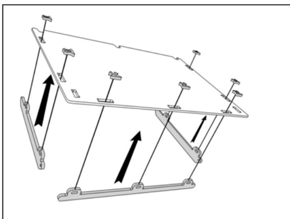
15 , Fixez la traverse frontale du nichoir et les deux traverses latérales sur le pondoir du pondoir, dont la face verte doit être orientée vers le haut, à l'aide des éléments suivants
