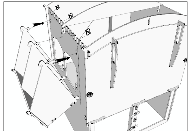
14 , Installez le pondoir en insérant d'abord les pattes en L dans les trous inférieurs de la paroi latérale droite, puis en inclinant le nichoir pour faire passer les trois pattes supérieures dans leurs trous, avant de les fixer à l'intérieur du poulailier avec 2 goupilles.
