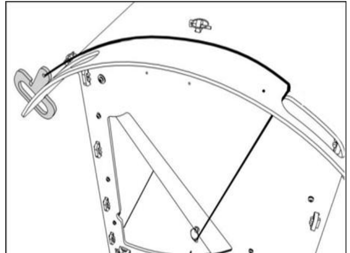
20, NUR BEI MANUELLER TÜR: Binden Sie ein Ende der Schnur an den geteilten Ring in der Vordertür und das andere Ende an das kleine Loch im Türgriff. Die Schnur sollte durch den Schlitz im Griff verlaufen. Stellen Sie die Länge der Schnur so ein, dass der Griff bei vollständig angehobener Tür gerade noch an der Kante des gegenüberliegenden Haltegriffs oder an der Dachkante einhakt.
