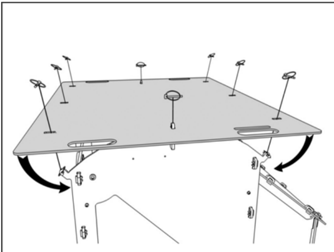
19, Befestigen Sie das Dach mit Klappsplinten. Befestigen Sie zuerst die Mitte und biegen Sie dann die Seiten über die verbleibenden Laschen
