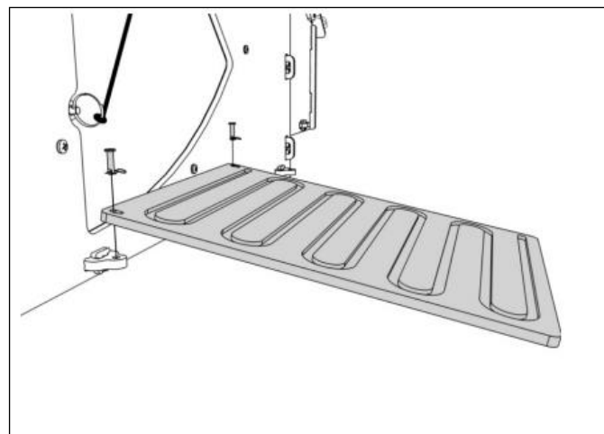
21 Montieren Sie die Rampe auf den beiden Laschen (Vorderseite) mit 2 x 25 mm Clevis Pins und 2 x RClips. Es neigt sich unter seinem eigenen Gewicht zum Boden.
