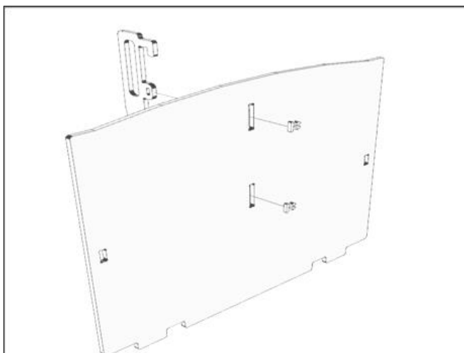
10 Fixez la poignée de la porte arrière sur le côté texturé de la porte arrière à l'aide de 2 clips Pi. Le crochet en forme de L sur le dessus de la poignée indique le haut.
