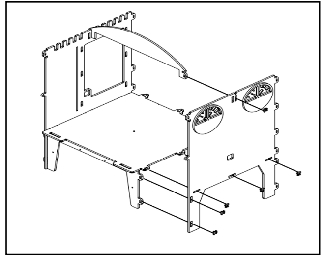
7 Fixez la paroi latérale (avec les événements) à la base et aux pieds, puis fixez le support de toit aux fentes centrales supérieures des murs à l'aide de 6 x Pi clips.
