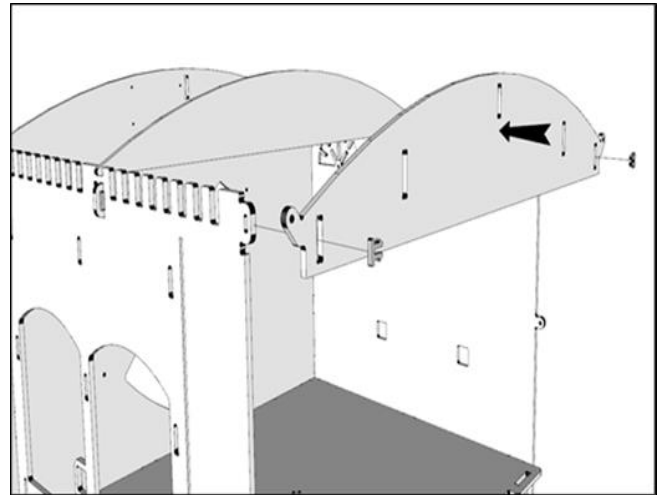
9 Fixez le support de toit arrière aux deux pattes supérieures à l'aide de 2 x Pi Clips.
