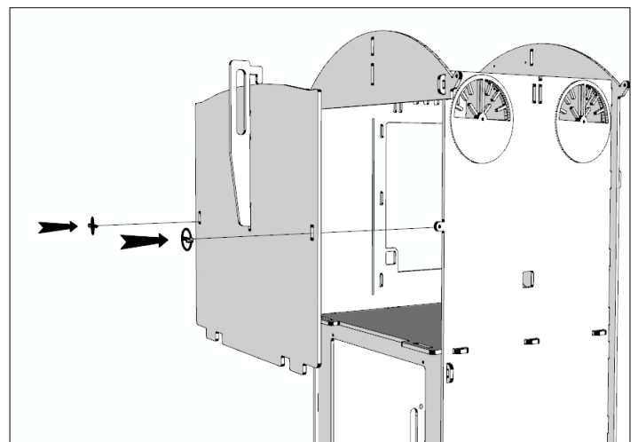
11 Installez la porte arrière à l'aide de deux goupilles de fixation. (Lors du montage, posez d'abord le bas de la porte arrière dans les fentes de la base, puis poussez la porte sur les pattes latérales et faites glisser la poignée de la porte arrière vers le bas pour verrouiller. Verrouillez-la avec des goupilles.
