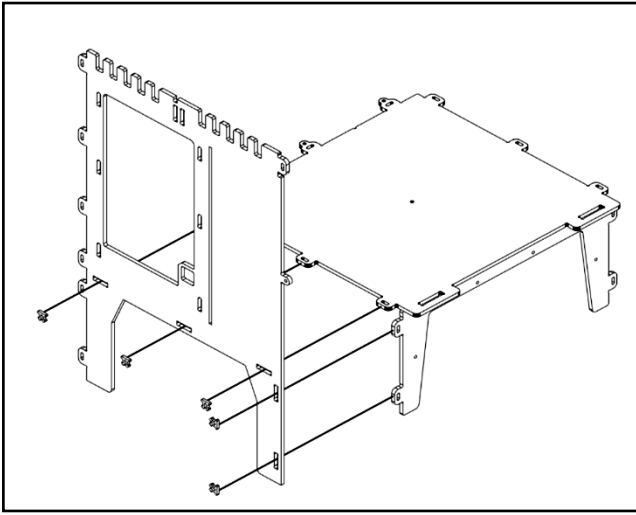
6 Ajustez la paroi latérale au plancher et au pied arrière à l'aide de clips Pi. Le côté lisse côté intérieur.
