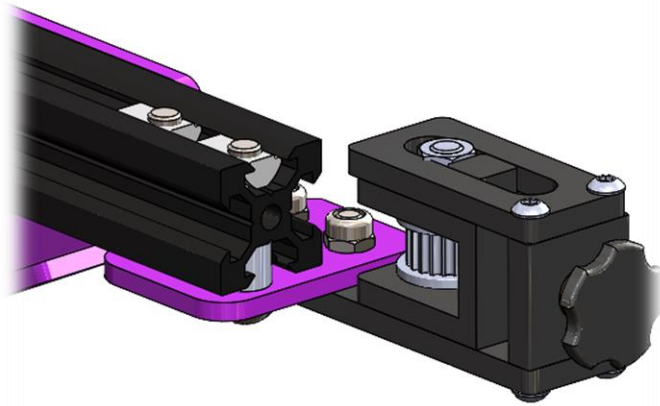
Figure 48 Left tensioner mount.
