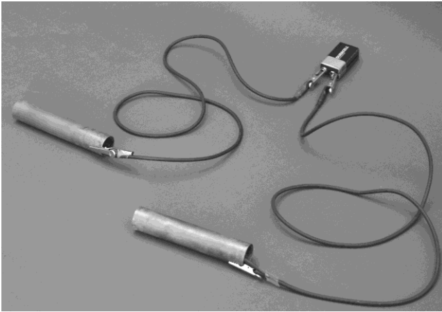
Fig. 5 Simple pulser
