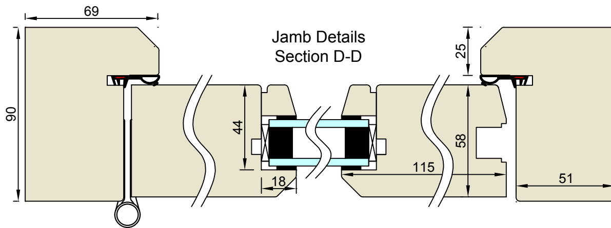
Option 1; Bevel Edge
