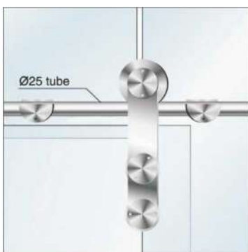
26602-25H ROD
