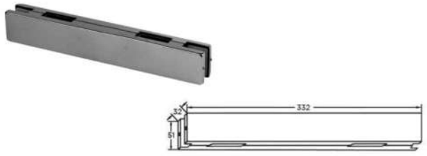
26201-D OVER PANEL DOUBLE DOOR STRIKE
