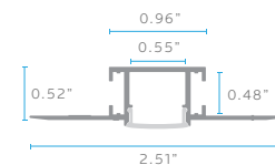
DIMENSIONS
