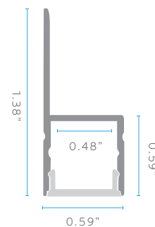
DIMENSIONS
