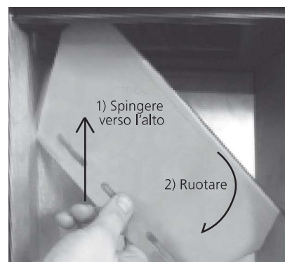
Fig. 17: estrazione del battifiamma
