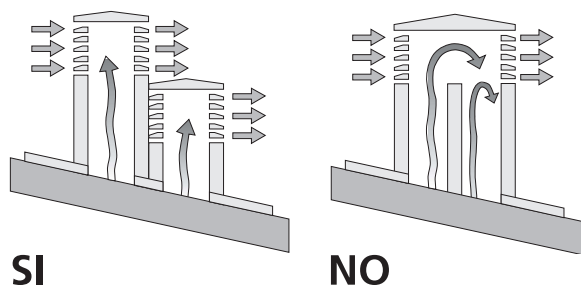
Fig. 5: caratteristiche del comignolo
