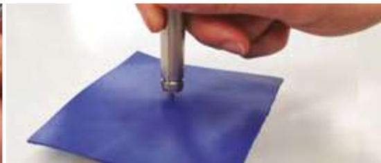
OUTIL DE POSE POUR RIVETS À MATER
