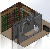
吊顶式安装
