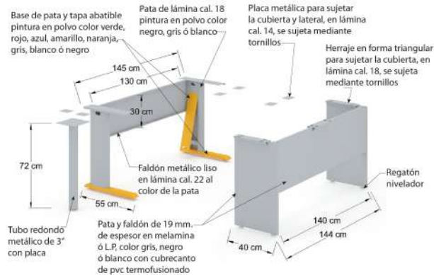
Especificación gráfica de chasis línea Moville Space Plus (PGDSS24)
