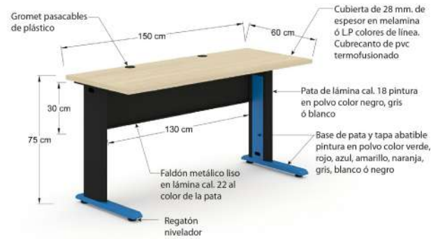
Especificación gráfica de cubierta línea Moville Space Plus (ESPSS18)
