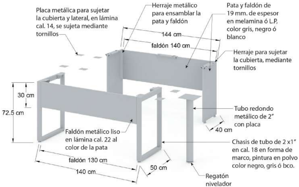
Especificación gráfica de chasis línea Movable operativa (PGDMT24)
