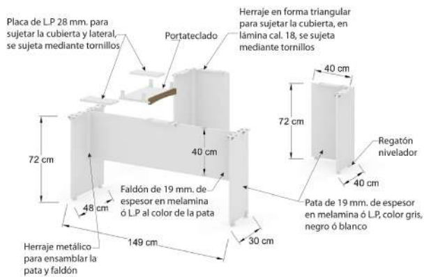
Especificación gráfica de chasis línea Qualium (LPAQEJE1)
