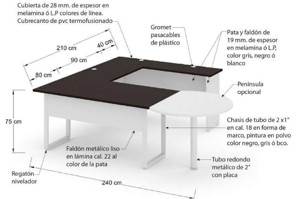
Especificación gráfica de cubierta línea Movable operativa (PGDMT24)
