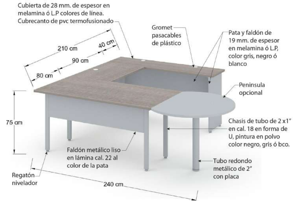
Especificación gráfica de cubierta línea Movable operativa (PGD1MT24)
