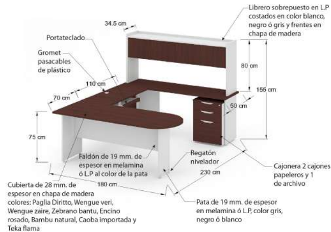
Especificación gráfica de cubierta línea Qualium Chapa (LPAQEJE1)
