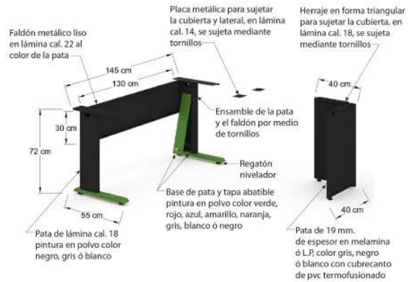
Especificación gráfica de chasis línea Moville Space Plus (PGDSS24)
