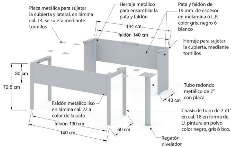
Especificación gráfica de chasis línea Movable operativa (PGD1MT24)
