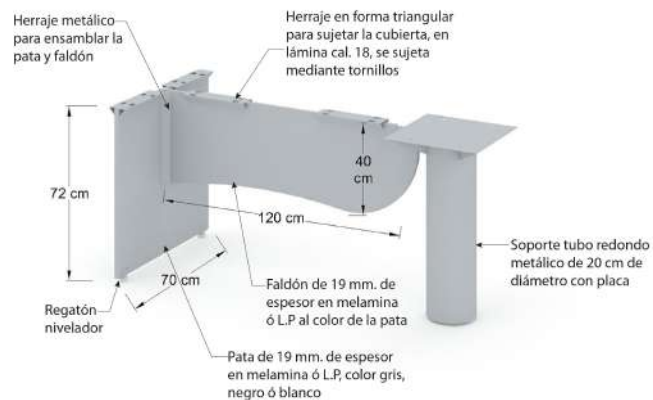
Especificación gráfica de chasis línea Qualium (PBQUA818)
