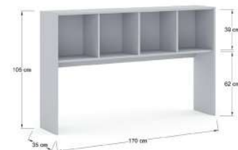
ALBR1735 Librero abierto fabricado en laminado pástico 19mm, con 4 nichos, sin forro en la parte baja. Para credenza de 180 cm.
