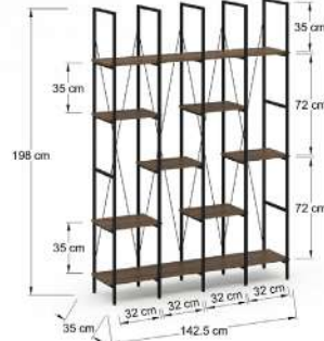
NS142 Librero de 4 entrepaños en mdf 15 mm., estructura metálica, tubular cuadrado de 3/4" y cruceta en redondo de 1/4".
