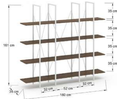
NS180 Librero de 4 entrepaños en mdf 15 mm., estructura metálica, tubular cuadrado de 3/4" y cruceta en redondo de 1/4".
