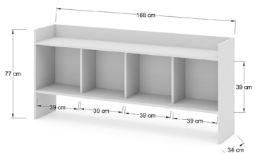
EXLB1634 Librero abierto fabricado en laminado pástico 19mm, con 4 nichos, sin forro en la parte baja.
