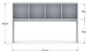
ALBR1735 Librero abierto fabricado en laminado pástico 19mm, con 4 nichos, sin forro en la parte baja. Para credenza de 180 cm.
