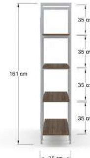
NS180 Librero de 4 entrepaños en mdf 15 mm., estructura metálica, tubular cuadrado de 3/4" y cruceta en redondo de 1/4".
