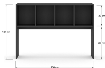
ALBR1535 Librero abierto fabricado en laminado pástico 19mm, con 4 nichos, sin forro en la parte baja. Para credenza de 160 cm.
