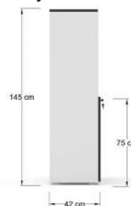
Librero metálico con 3 entpaños de 80x42x145 cm. con puertas inferiores. y cubierta en l.p. incluye chapa.
