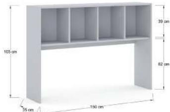
ALBR1535 Librero abierto fabricado en laminado pástico 19mm, con 4 nichos, sin forro en la parte baja. Para credenza de 160 cm.
