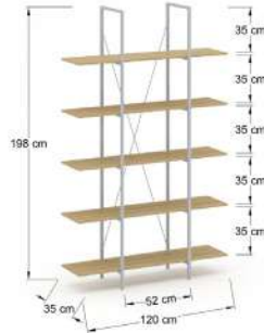
NS120 Librero de 5 entrepaños en mdf 15 mm., estructura metálica, tubular cuadrado de 3/4" y cruceta en redondo de 1/4".
