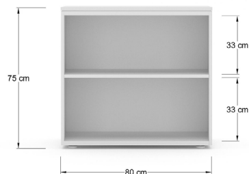
Librero metálico con 1 entpaño de 80X40X75 cm.
