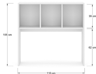
ALBR1035 Librero abierto fabricado en laminado pástico 19mm, con 3 nichos, sin forro en la parte baja. Para credenza de 120 cm.
