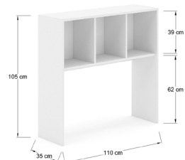
ALBR1035 Librero abierto fabricado en laminado pástico 19mm, con 3 nichos, sin forro en la parte baja. Para credenza de 120 cm.
