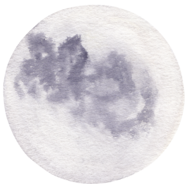
Pleine lune
