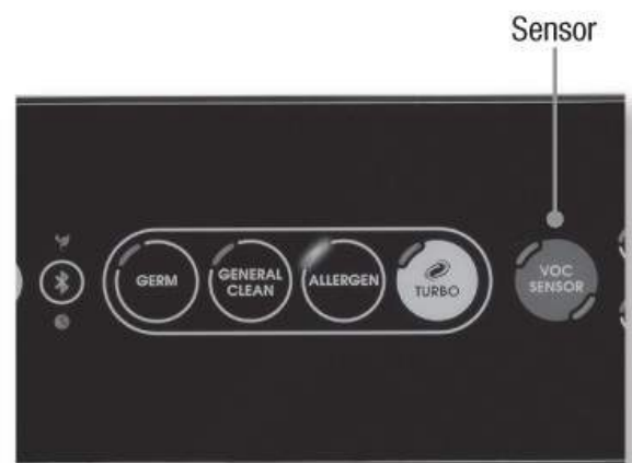
Fig. 8 VOC Function
