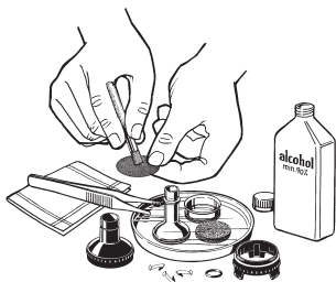
Handamtige reiniging isopropylalcohol (70 %) of reinigingsmiddel
