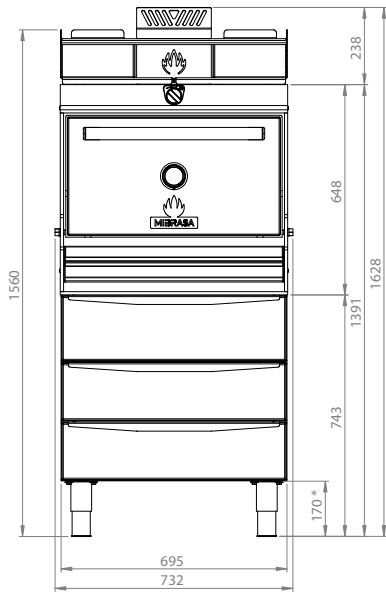
Vue frontale
