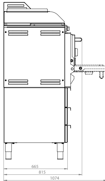
Vue latérale
