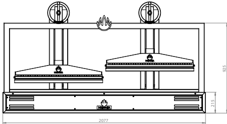
Vue frontale
