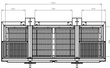
Vue supérieure
