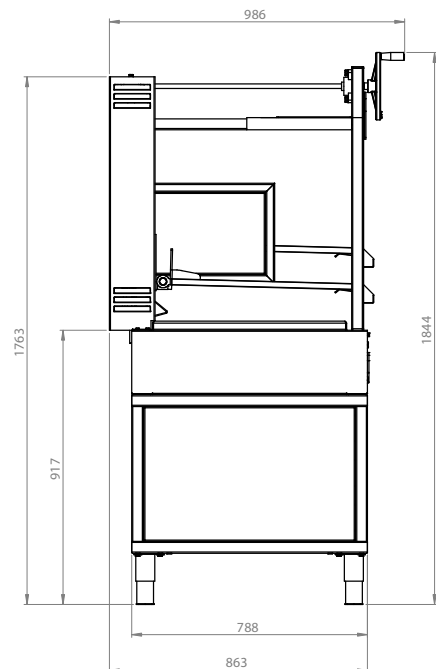
VUE LATÉRALE
