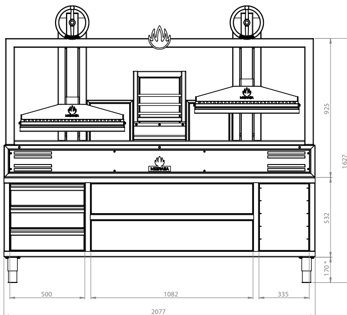
VUE FRONTALE
