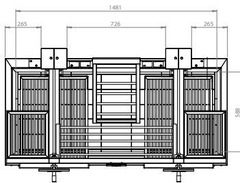
Vue supérieure
