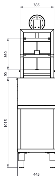
VUE LATÉRALE
