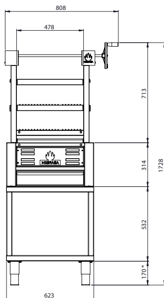
VUE FRONTALE
