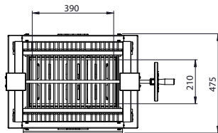
Vue supérieure
