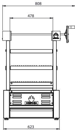
Vue frontale
