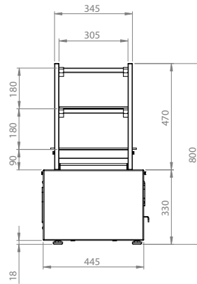
Vue latérale
