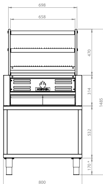
VUE FRONTALE
