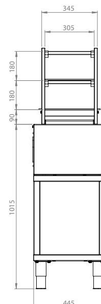
VUE LATÉRALE
