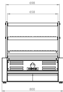
Vue frontale
