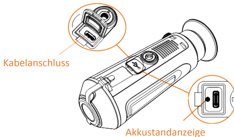
Abbildung 2-1 Kabelanschluss
