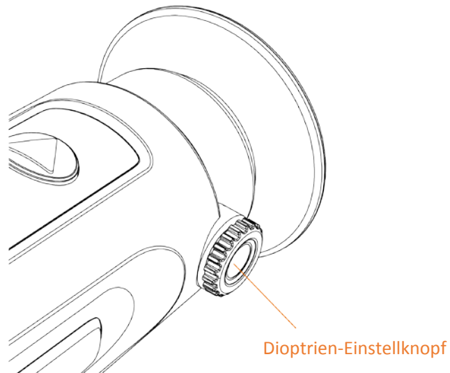
Abbildung 3-2 Dioptrien einstellen
