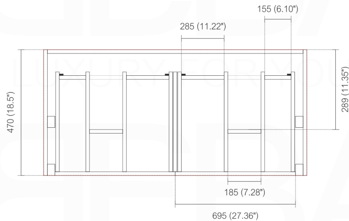
TOP ELEVATION
