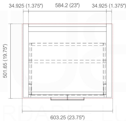
. TOP ELEVATION
