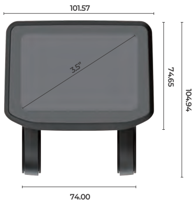
Vooraanzicht
