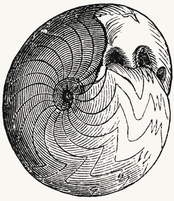
GONIATITES
