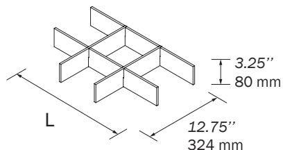
Organizer for wood drawer, Carbon-TX Organisateur pour tiror en bois, Carbon-TX
