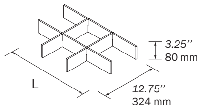
Organizer for wood drawer, Carbon-TX Organisateur pour tiroir en bois, Carbon-TX
