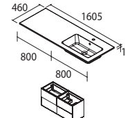
63"/1605 mm Left/Gauche (32"+32"/800+800 mm)
