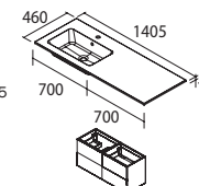
55"/1405 mm Right/Droite (28"+28"/700+700 mm)
