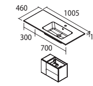
40"/1005 mm Left/Gauche (12"+28"/300+700 mm)
