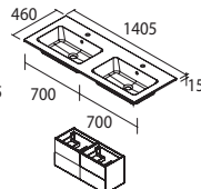
55"/1405 mm 2 units/2 unités
