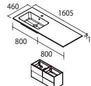
63"/1605 mm Right/Droite (32"+32"/800+800 mm)
