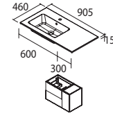
36"/905 mm Right/Droite (24"+12"/600+300 mm)
