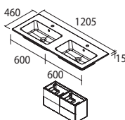
48"/1205 mm 2 units/2 unités
