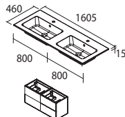
63"/1605 mm 2 units/2 unités
