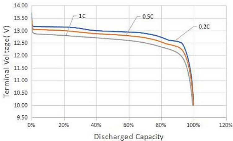
バッテリーの放電特性
