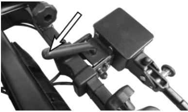
Bild 17: Abklappmechanismus
