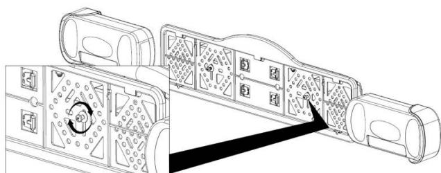
Figura 5: Montaggio portatarga
