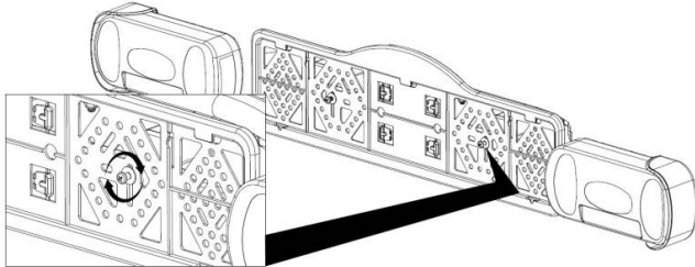
Bild 5: Montage Kennzeichenhalter
