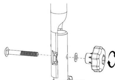
Bild 3: Festschrauben U-Bügel
