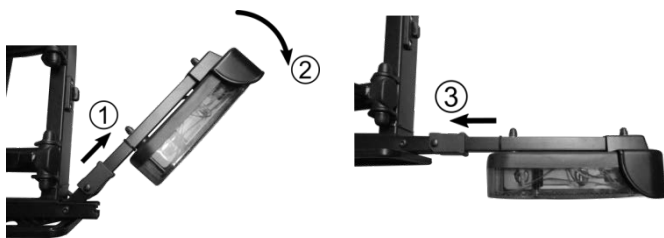
Bild 12: Verriegelung Leuchtenträger
