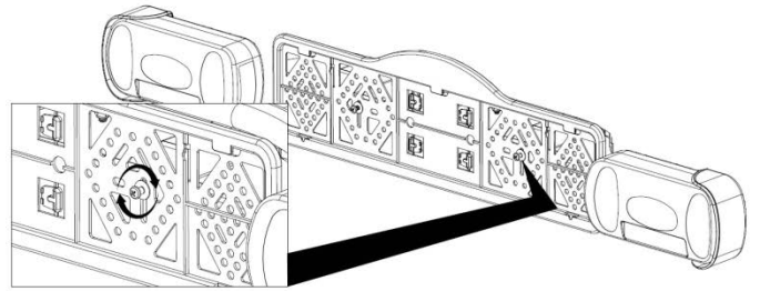
Bild 5: Montage Kennzeichenhalter
