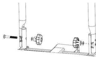
Figure 2 : Montage de l'étrier en U
