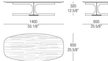
Petite Table semi-ovale avec plateau en bois
