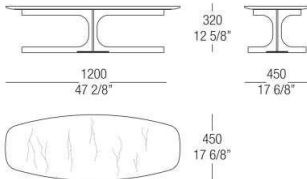
Petite Table semi-ovale avec plateau en marbre
