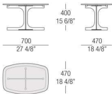
Petite Table semi-ovale avec plateau en verre
