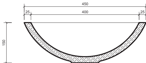
Sețiune Scara.1/10
