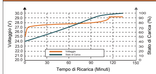
CURVA DELLO STATO DI CARICA (0.5C, 25°C)
