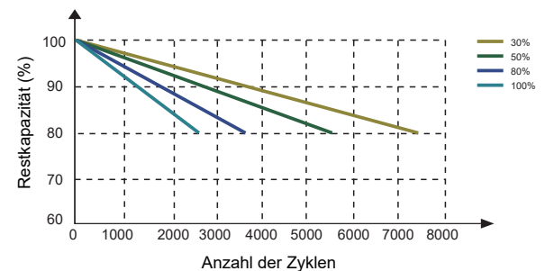
UNTERSCHIEDLICHE DOD-ENTLADUNGSZYKLUS-LEBENSKURVE
