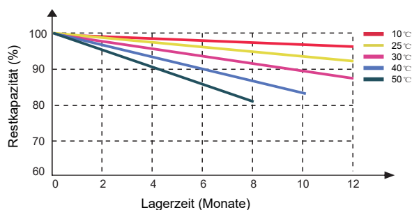
UNTERSCHIEDLICHE TEMPERATUR-SELBSTENTLADEKURVE
