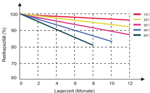
Unterschiedliche Temperatur-Selbstentladekurve
