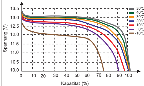
Unterschiedliche Temperatur-Entladungskurve (0.5C)
