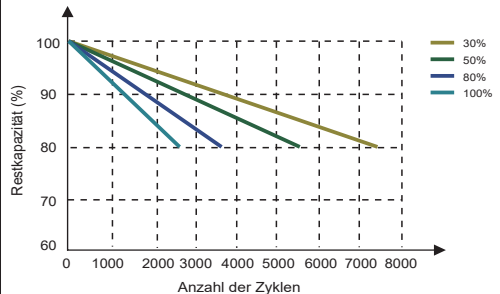
Unterschiedliche DOD-Entladungszyklus-Lebenskurve
