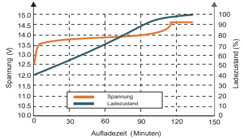
Ladezustandskurve (0.5C, 25°C)
