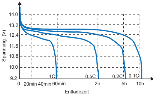
Entladekurve mit unterschiedlicher Rate (25°C)
