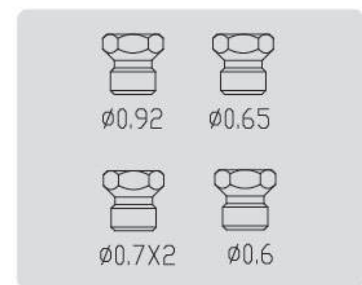
液化石油气喷嘴 (5)
