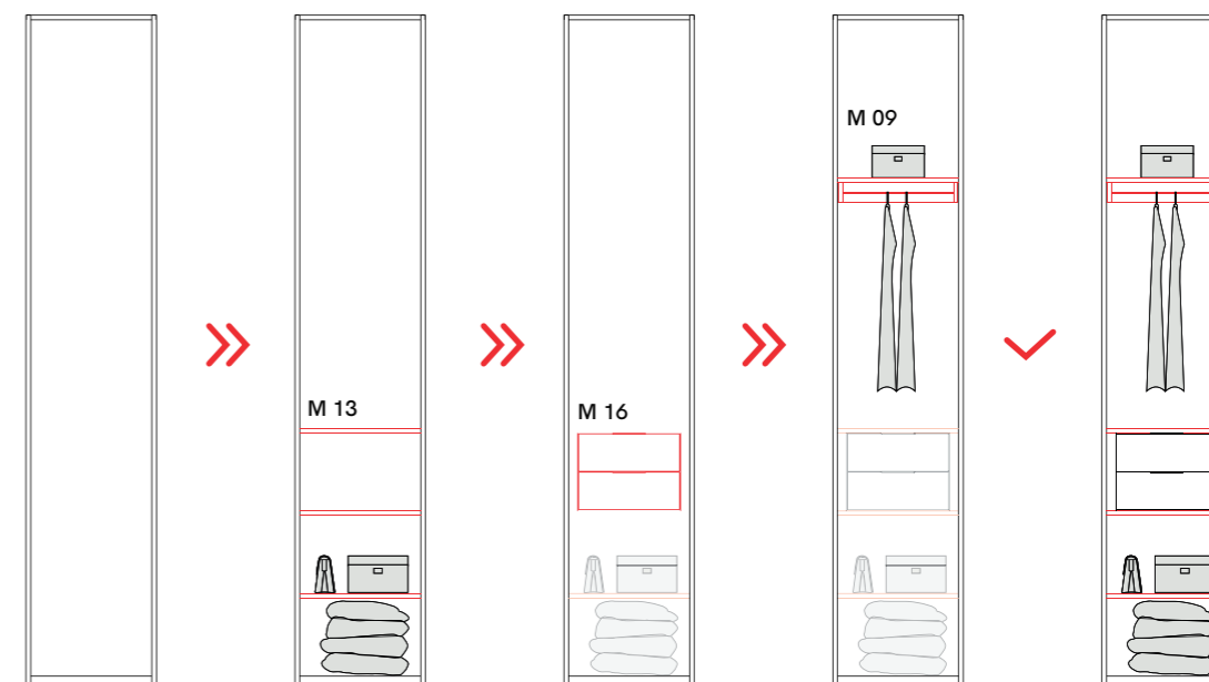
G 01 ALFA Корпус
